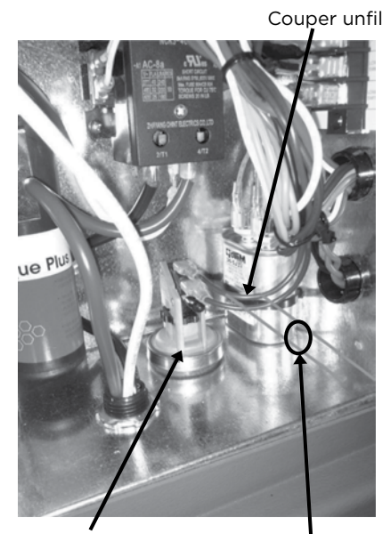
L'interrupteur de Pression 2 Câbles de base du panneau d'accès
